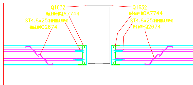
武汉学院实训楼幕墙JD-07
