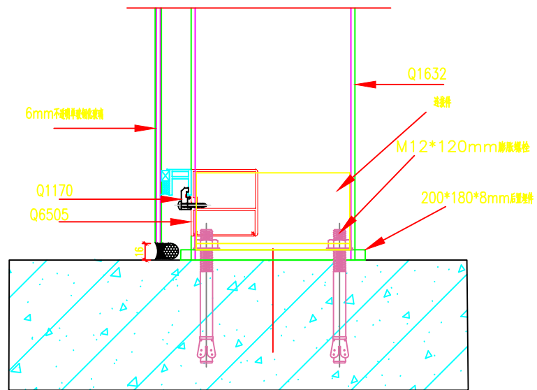
武汉学院实训楼幕墙JD-04
