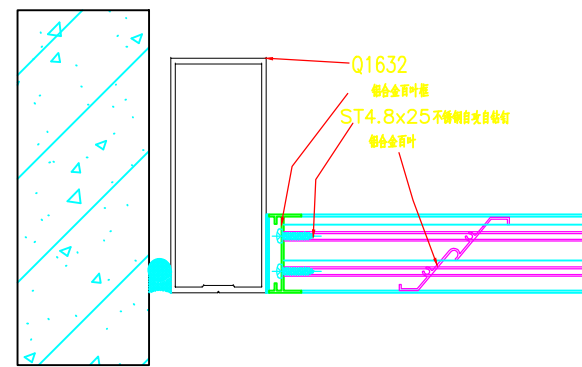
武汉学院实训楼幕墙JD-06
